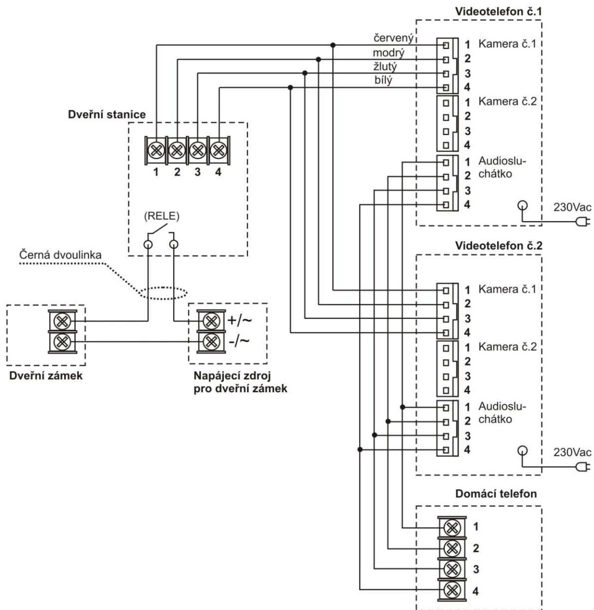
Schéma č.4 – Zapojení jedné dveřní stanice, dvou videotelefonů a jednoho domácího telefonu. Mezi oběma videotelefony a domácím telefonem je funkční interkomová komunikace
